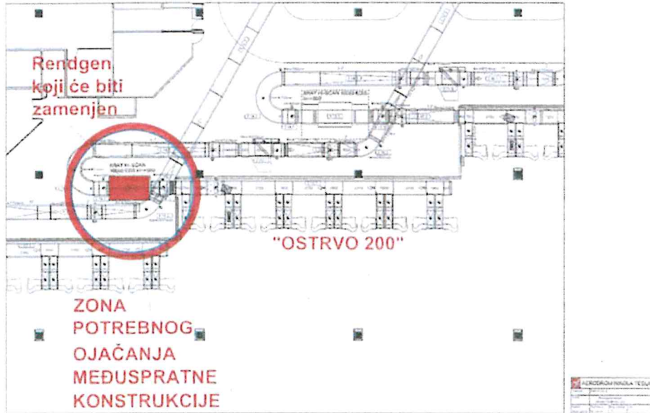
PRIZEMLJE TERMINALA 2 I ZONA OJAČANJA MEĐUSPRATNE KONSTRUKCIJE "OSTRVO 200"
