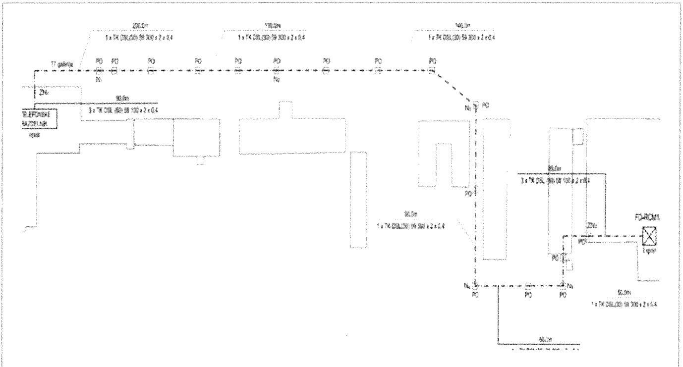
Сл.2. Траса спојног паричног кабла између главне аеродромске зграде и зграде РЦМ-а
