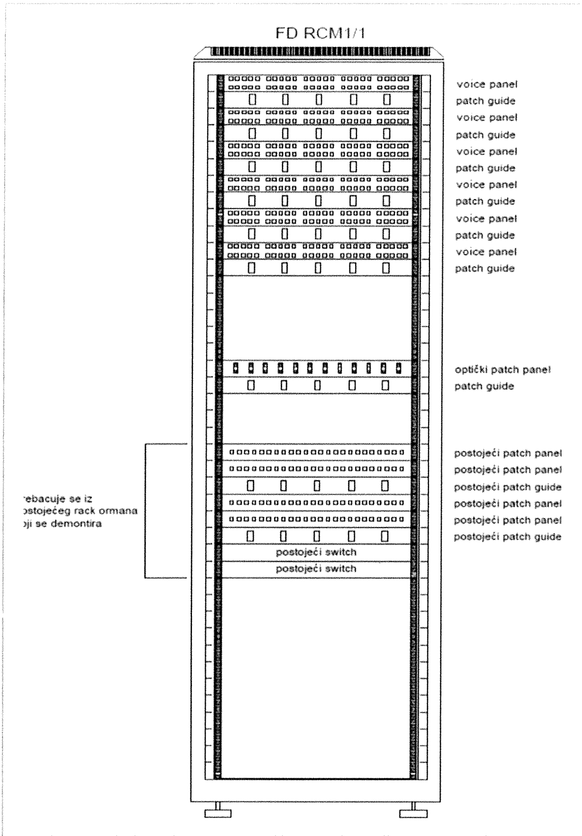
Сл. 4. Начин уређења новог рек ормана ФД РЦМ1/1, укључујући пребацивање опреме из постојећег рек ормана.
