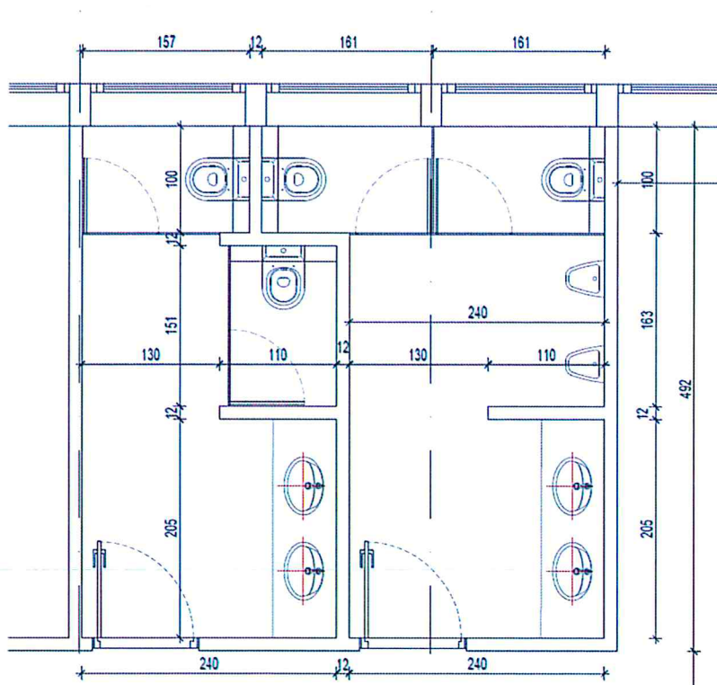
цртеж 2. планирано стање мокрог чвора
