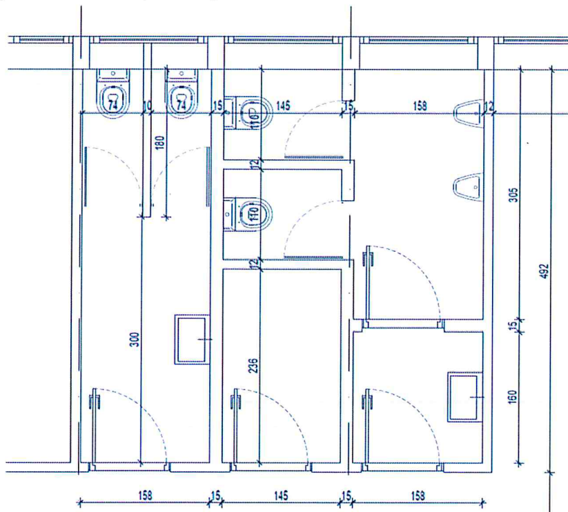
б) цртеж 1. постојеће стање мокрог чвора
